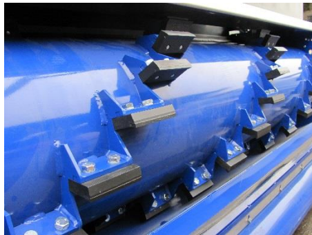
Terraplane® rotor
